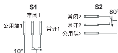
接线图
