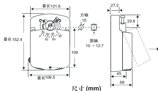
尺寸 (mm)
